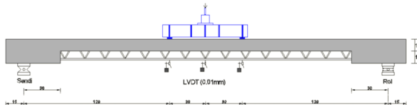
Gambar 1. Setup benda uji
