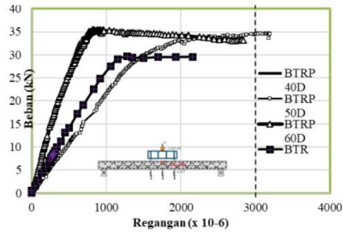
Gambar 5. Grafik hubungan beban dan regangan beton
