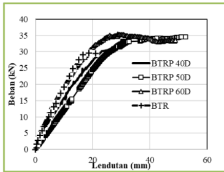
Gambar 4. Grafik hubungan beban dan lendutan
