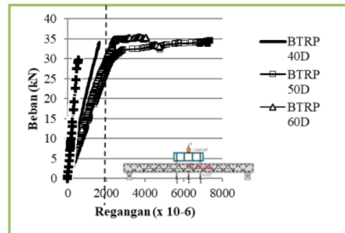
Gambar 6. Hubungan beban dan regangan tulangan utama
