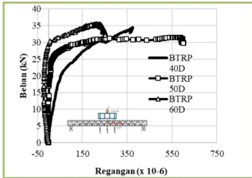
Gambar 7. Grafik hubungan beban dan regangan tulangan perkuatan
