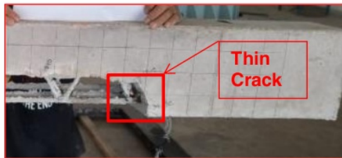
Gambar 11. Pola retak balok BTRP 60D
