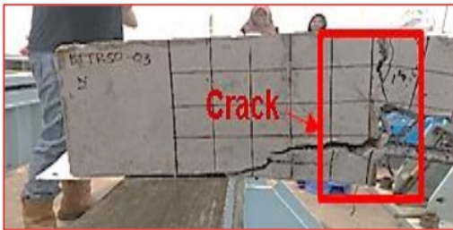
Gambar 8. Pola keruntuhan balok BTR
