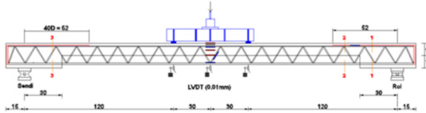
Gambar 2. Tampak depan benda uji
