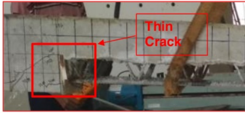
Gambar 10. Pola retak balok BTRP 50D
