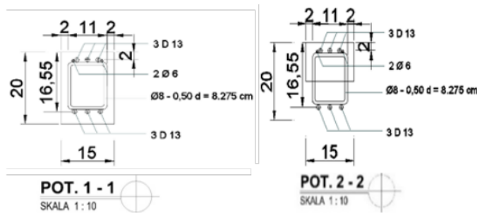
Gambar 3. Potongan benda uji
